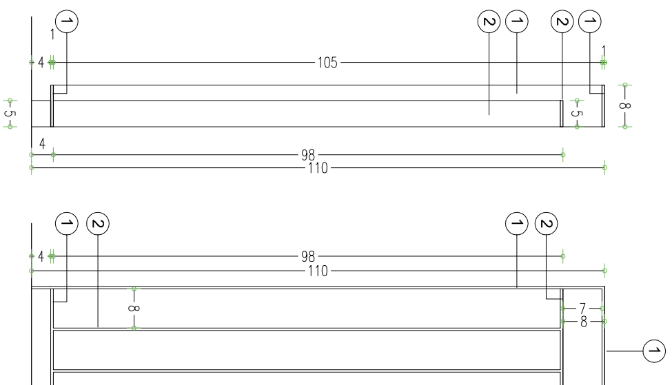
PRZEKRÓJ 1:10
